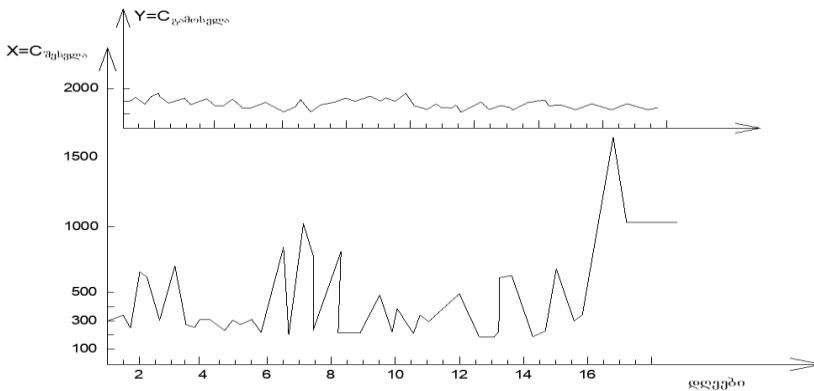
ნახ. 1. ელექტრომარილგამომცლელი დანადგარის შესასვლელში და გამოსასვლელში მარილების კონცენტრაციის შემოფოთებათა გრაფიკი
