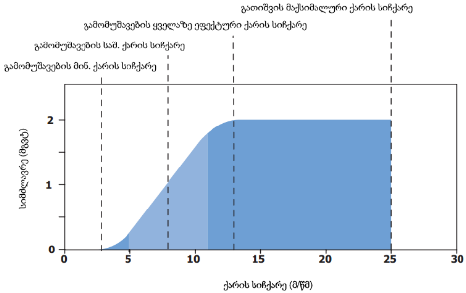
დანართი 7. ქარის ტურბინის სიმძლავრის ტიპური მრუდი [8];
