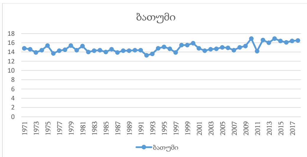
ნახ. 1. ბათუმის თერმული რეჟიმის მრავალწლიური მსვლელობა
