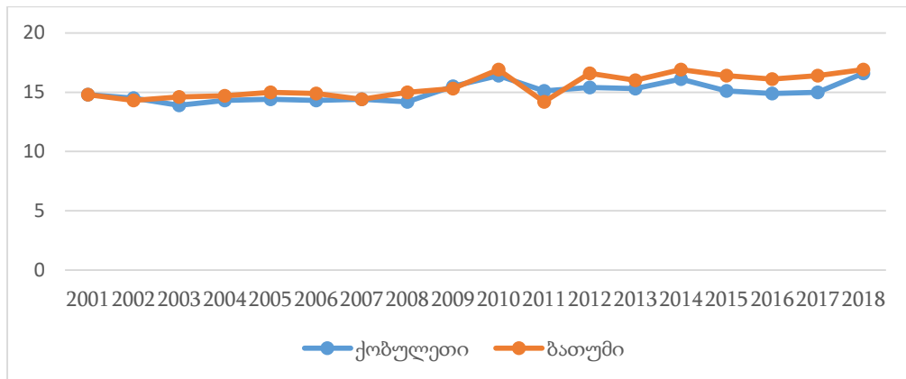
ნახ. 2. ბათუმისა და ქობულეთის საშუალო მრავალწლიური თერმული რეჟიმის მსვლელობა
