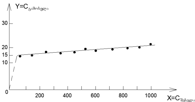
ნახ. 4. მარილის კონცენტრაციების დამოკიდებულება შესასვლელსა და გამოსასვლელს შორის
