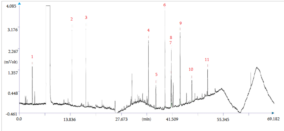
ნახ.1. ნავთობშლამის ორგანული ექსტრაქტის ქრომატოგრამა
