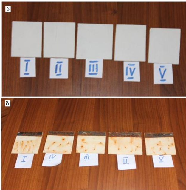
ნახ.2. დაფარული ფოლადის ნიმუშები: ა - გამოცდამდე; ბ - გამოცდის შემდეგ.
