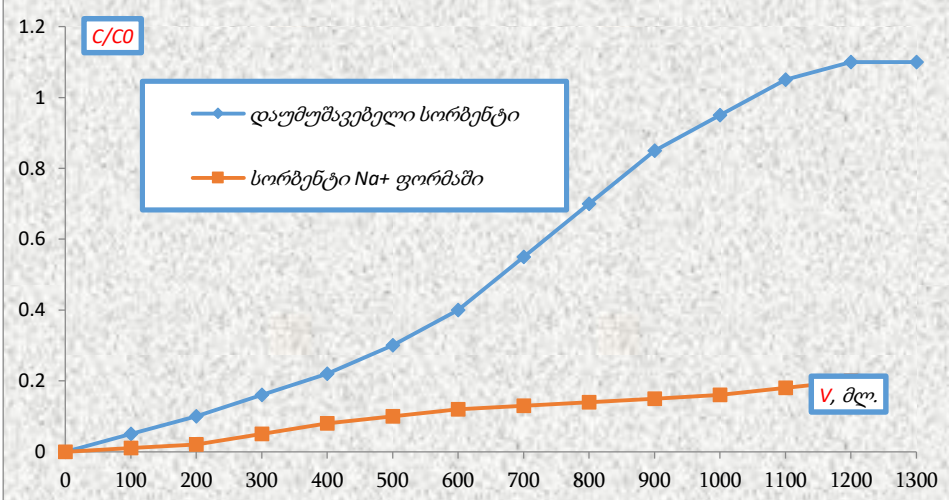
ნახ.9 ადსორბციის იზოთერმები \text{NH}_4\text{NO}_3 ხსნარიდან
