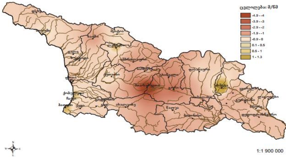
დანართი 8. ქარის საშუალო სიჩქარის წლიური მნიშვნელობების ცვლილება 2071-2100 წწ. და 1986-2010 წწ., [5].
