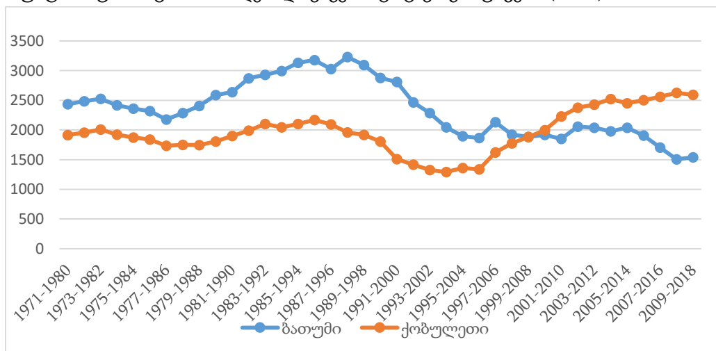
ნახ. 3. ბათუმისა და ქობულეთის იანვრის თვის ნალექების მცოცავი გრაფიკი იანვრის თვის ნალექებზე დაკვირვებამ ნათლად გვიჩვენებს, რომ 1971 წლიდან 2008 წლამდე პერიოდში, იანვარში ბათუმის ატმოსფერული ნალექების რაოდენობა ყოველთვის ჭარბობდა ქობულეთის ანალოგიურ მაჩვენებელს,
