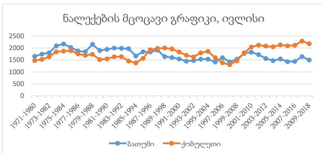
ნახ. 4. ბათუმისა და ქობულეთის იანვრის თვის ნალექების მცოცავი გრაფიკი
