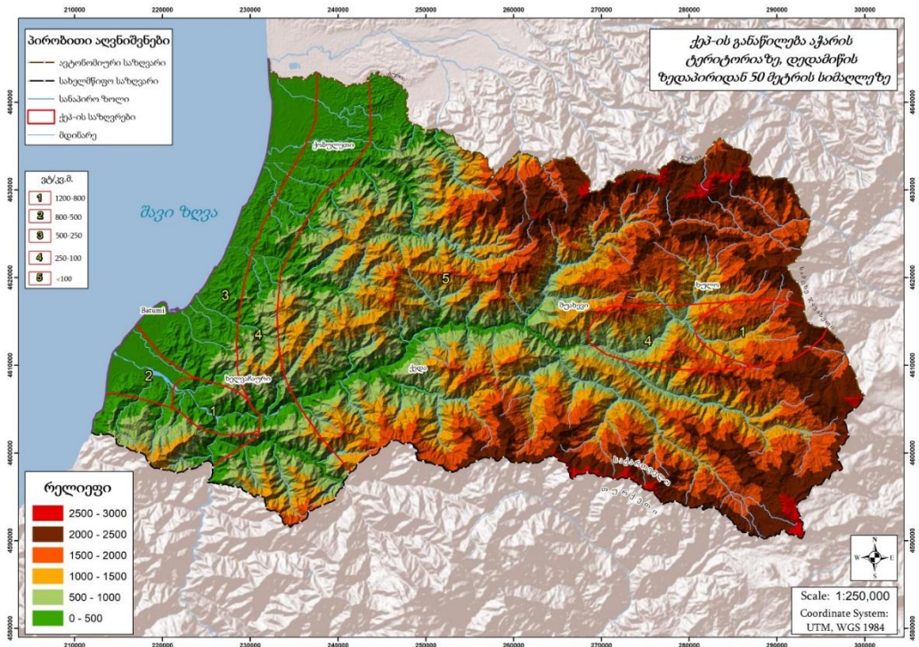
დანართი 5. ქარის ენერგეტიკული პოტენციალის განაწილება აჭარის ტერიტორიაზე, დედამიწის ზედაპირიდან 50 მეტრის სიმაღლეზე (ჩვენ მიერ შედგენილი რუკა, [4]-ის მონაცემების საფუძველზე);
