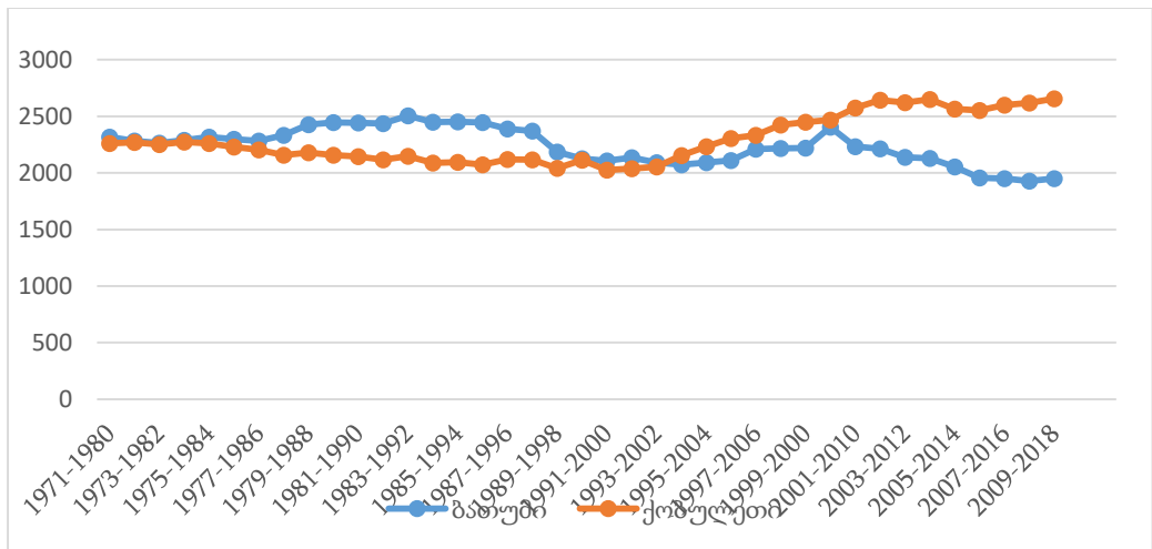
ნახ. 5. ნალექების მსვლელობის მრავალწლიური მცოცავი გრაფიკი
