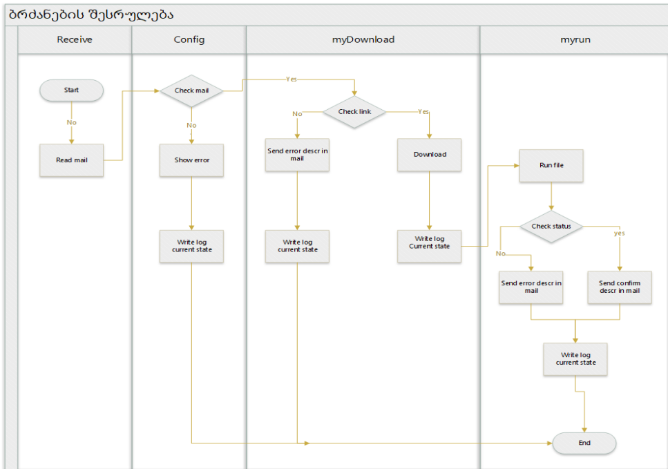
სურ. 1. სისტემური ბრძანების შესრულების ფუნქციონალური სქემა
