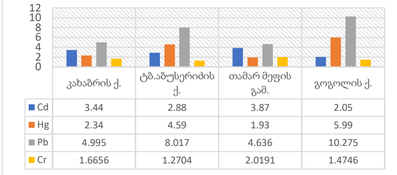
დიაგრამა N7. 2017 წლის მაისში სხვადასხვა უბანზე აღებული ნიმუშებში Cd, Hg, Pb, Cr კვლევის შედეგების შედარება.
